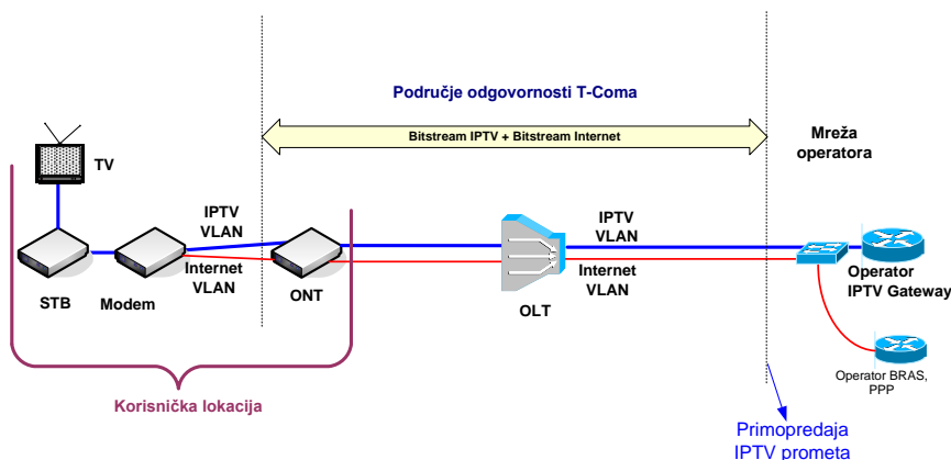
Slika 21. Veleprodajni širokopolasni pristup za pružanje IPTV usluge preko FTTH pristupa (GPON) na OLT razini
